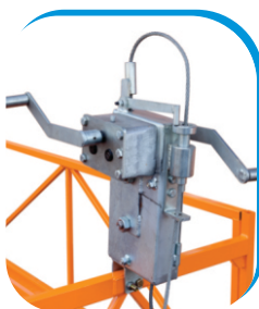
Tração Manual Manivela com Rolamento
